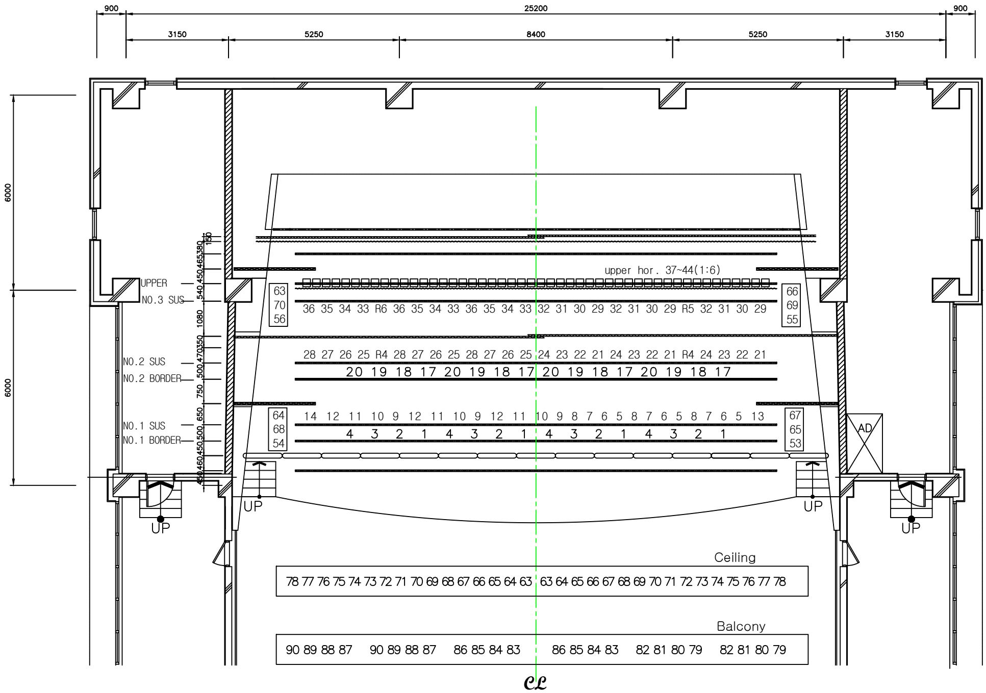
오정 아트홀 조명회로도
